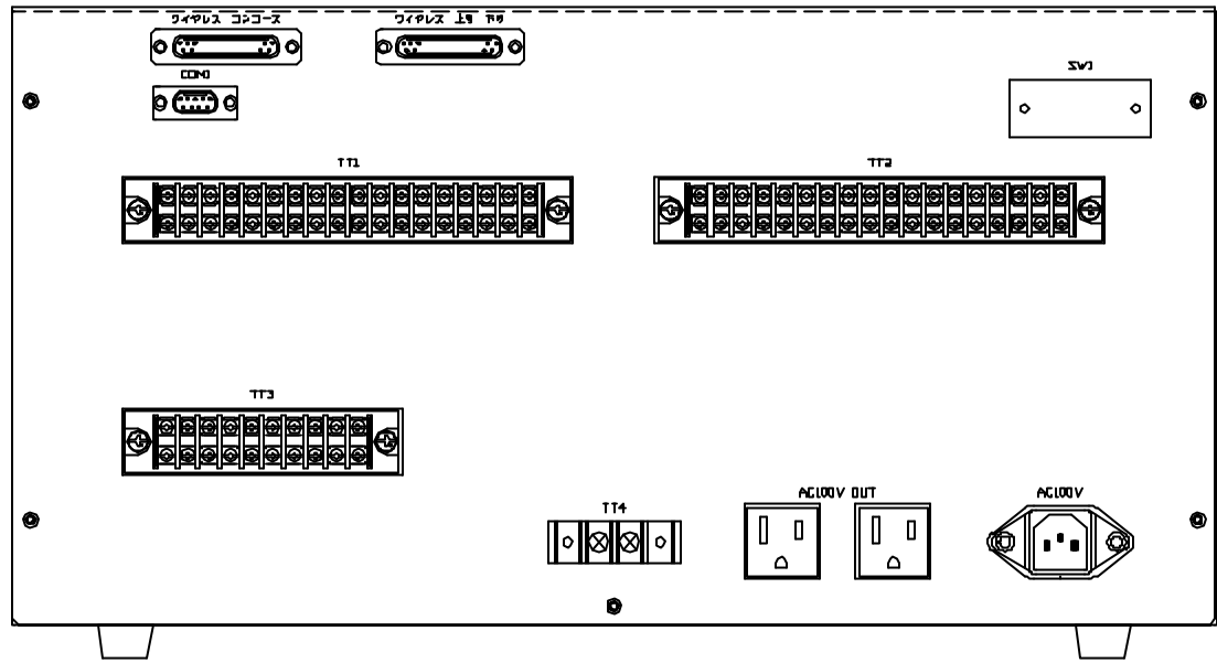
背面図
