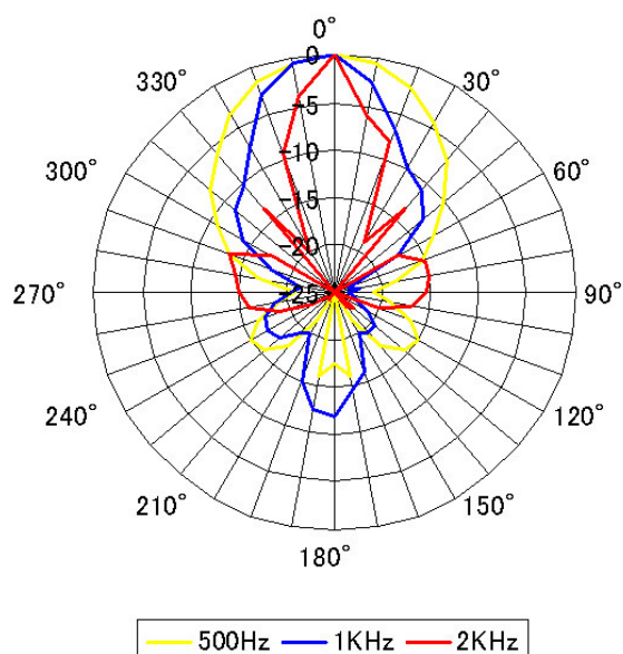
SNF-R4N水平指向性
