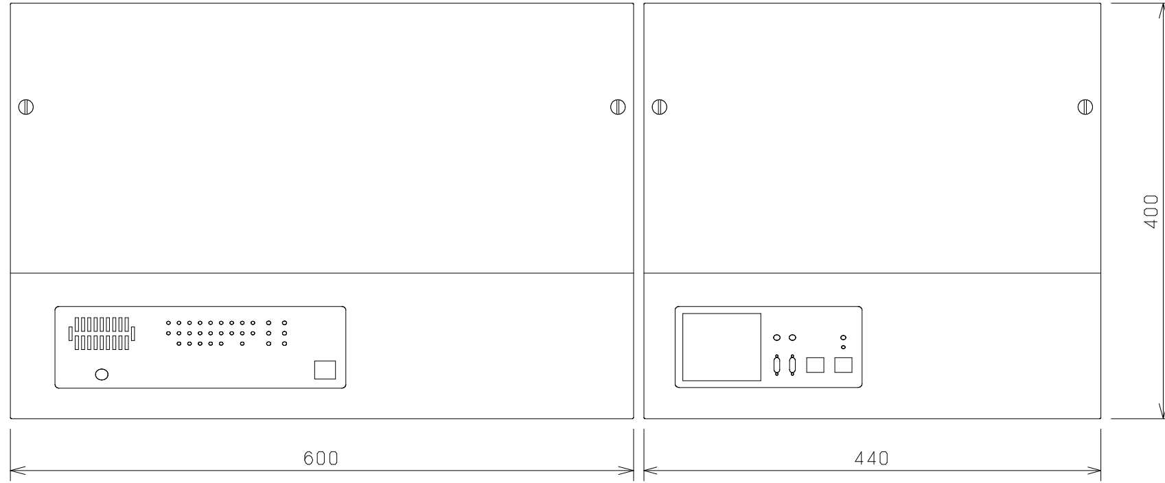
制御盤
