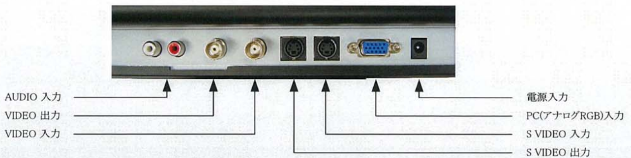
背面コネクター
